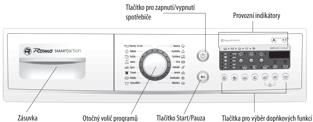
fig. 1 Ovládací panel
