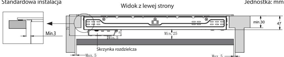
Standardowa instalacja
